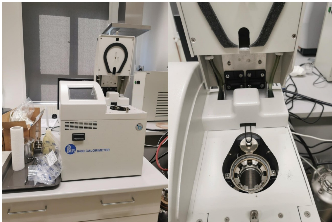
Zdj.3. Kalorymetr
