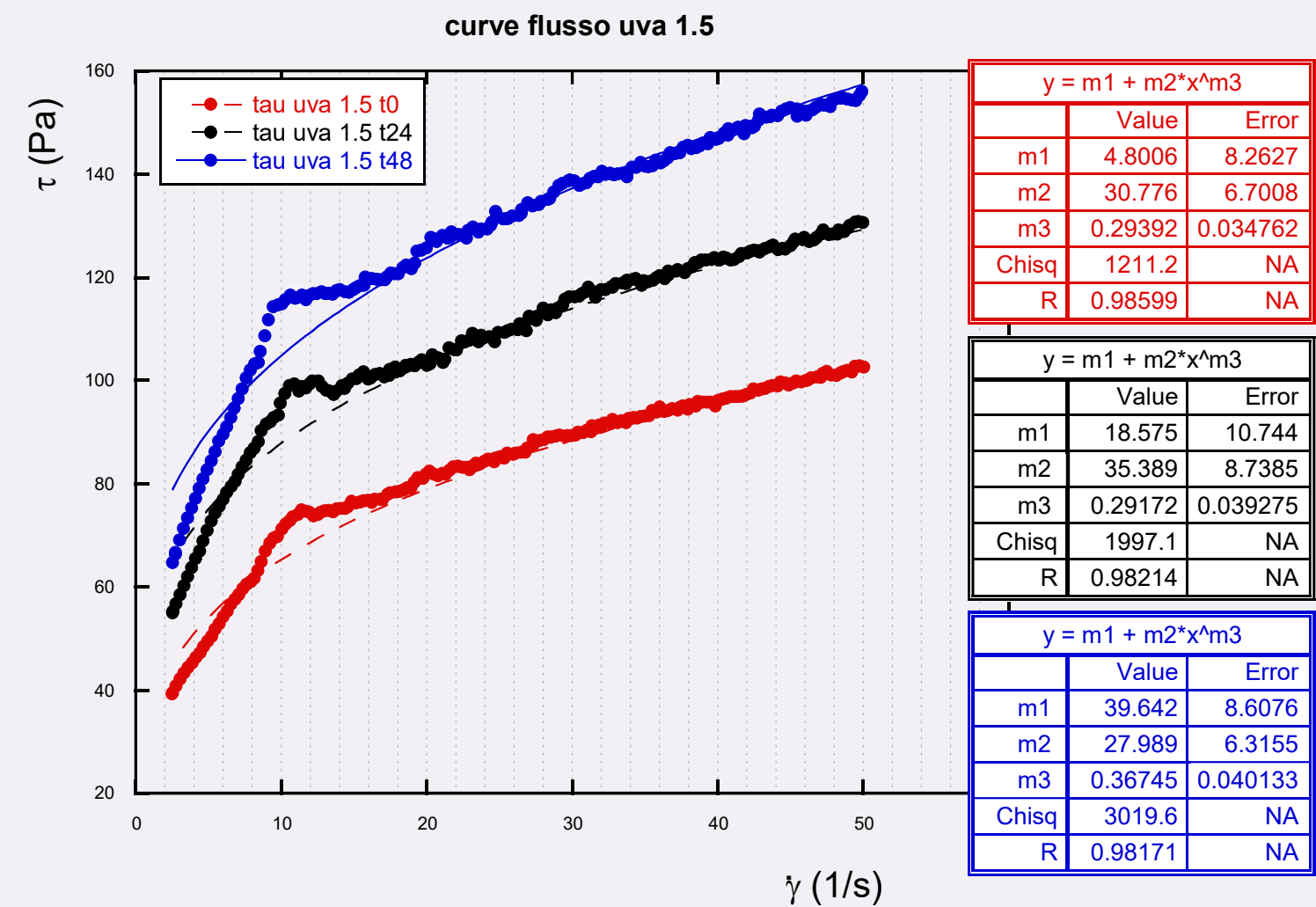
Rysunek 2 Wyniki wstępnej analizy reologii musu z dodatkiem proszku ze skórek i pestek z winogron 1,5g
