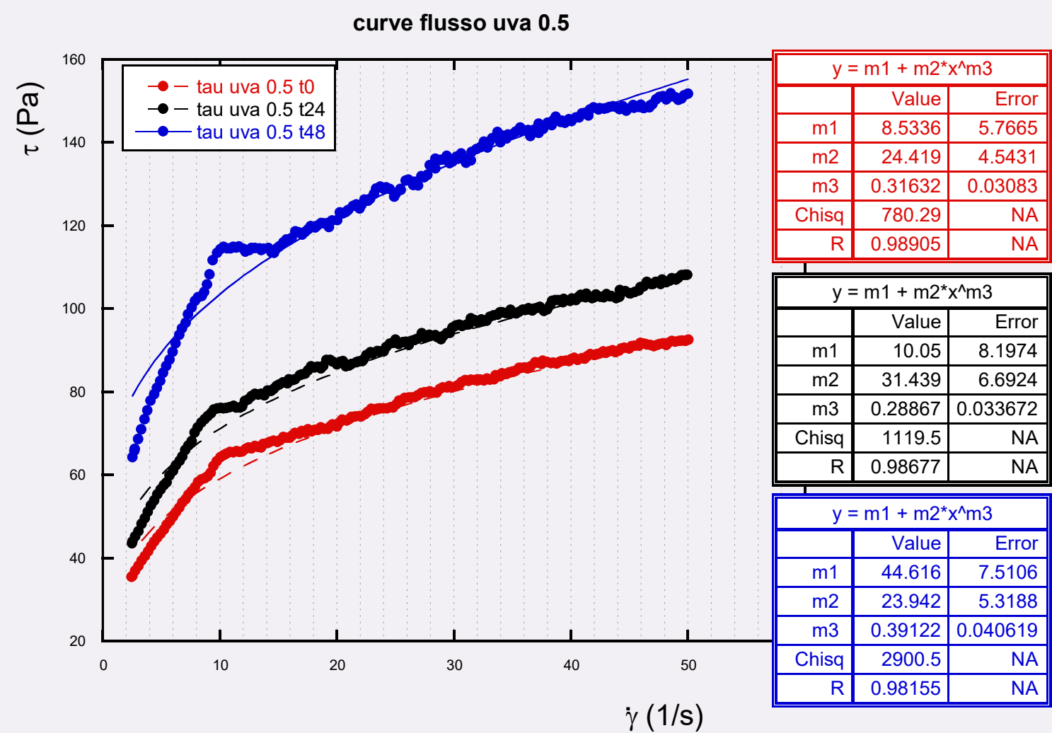
Rysunek 1 Wyniki wstępnej analizy reologii musu z dodatkiem proszku ze skórek i pestek z winogron 0,5g
